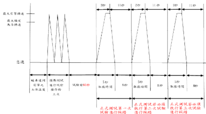
圖1 不透光率試驗過程圖
